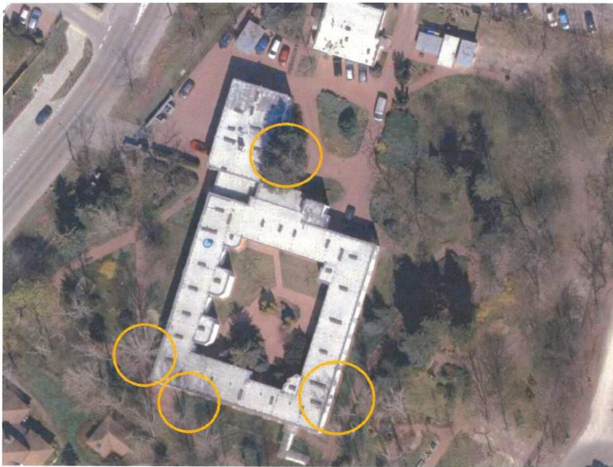
Rysunek 14 Rysunek poglądowy źródeł zacienienia budynku
