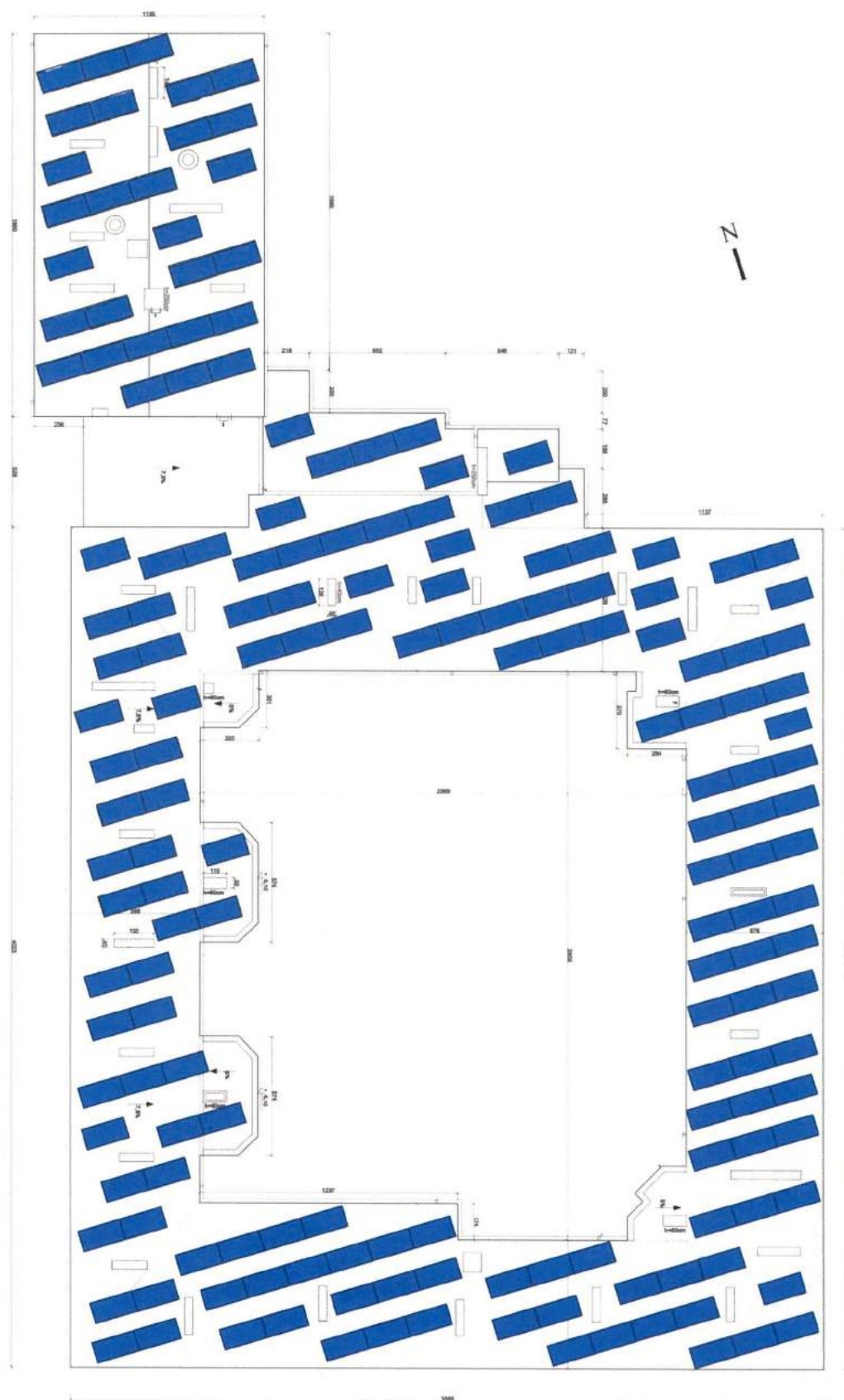
Rysunek 12 Proponowane rozmieszczenie paneli fotowoltaicznych na dachu budynku DPS
